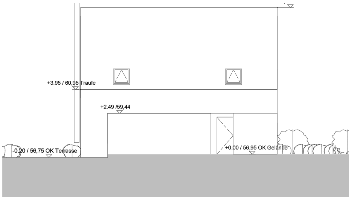
Ansicht Ost
