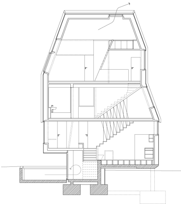
Schnitt A-A/ Section A-A
